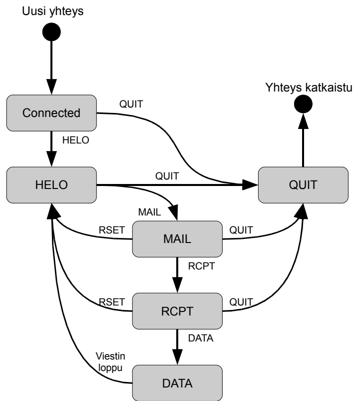
Kuva 3.1: SMTP-protokollan tilakone.
